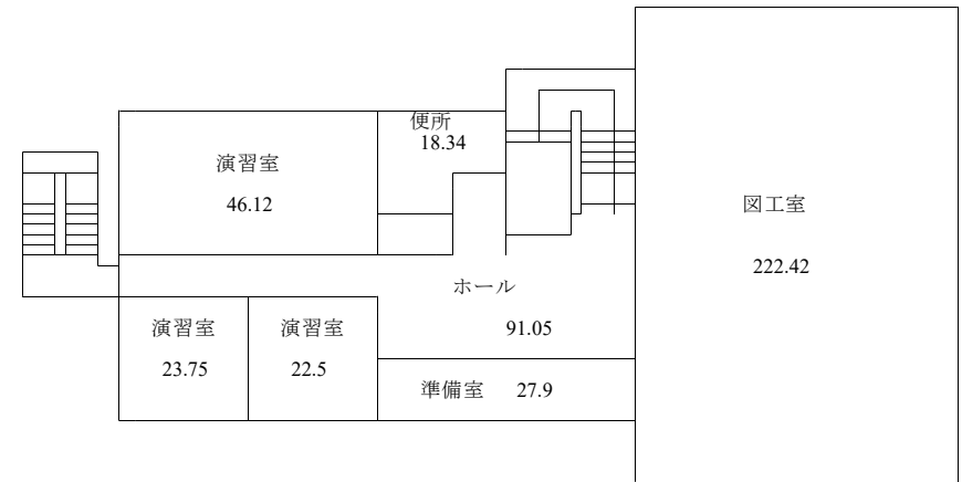
6号館 3階
