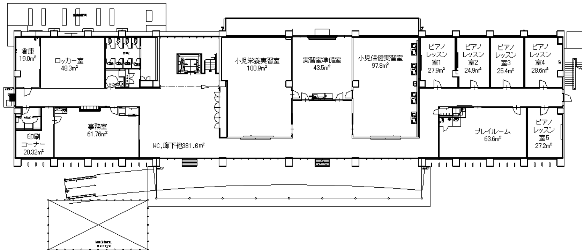
7号館 1階 平面図
